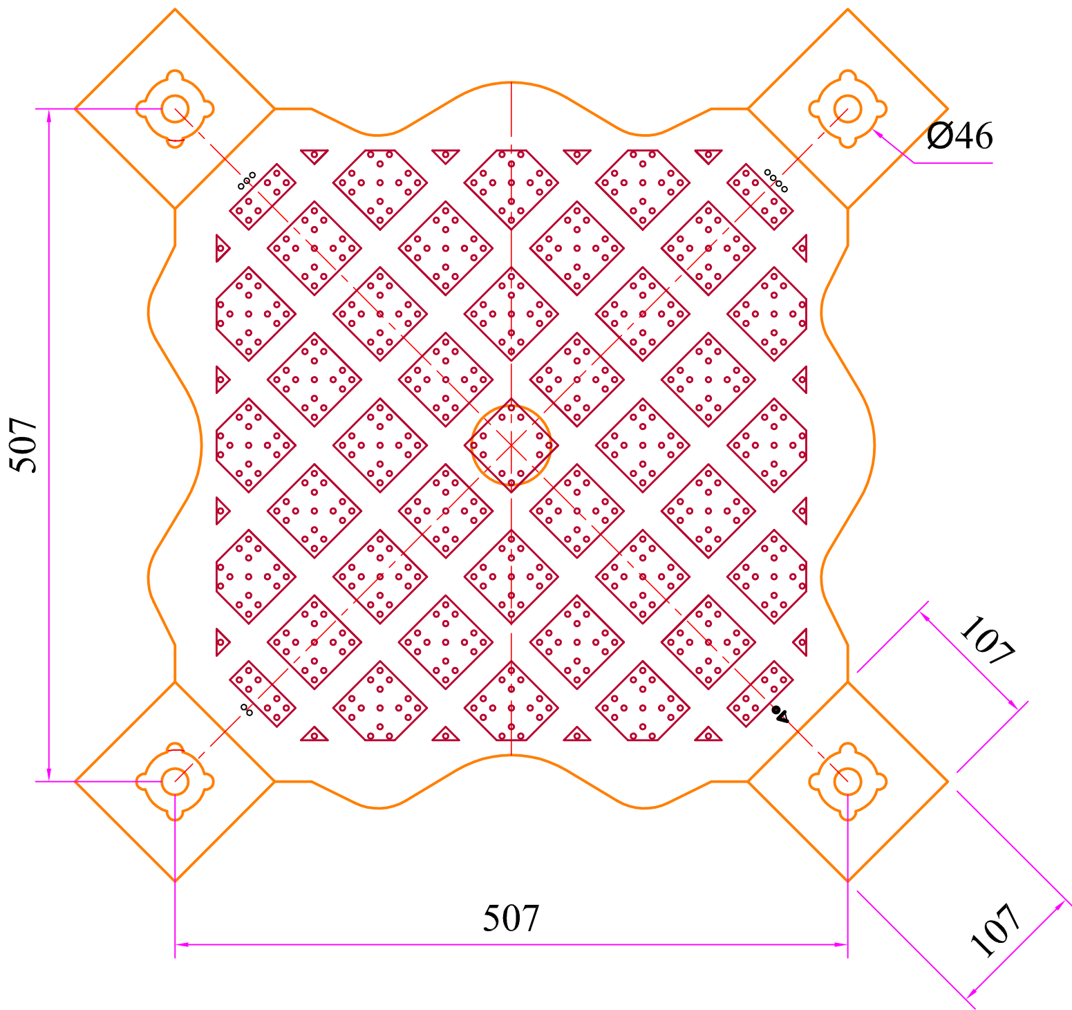
PHAO MODULE
